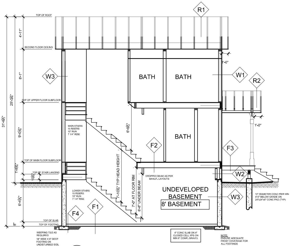
SECTION A-A SCALE: 3/16"=1'-0"
